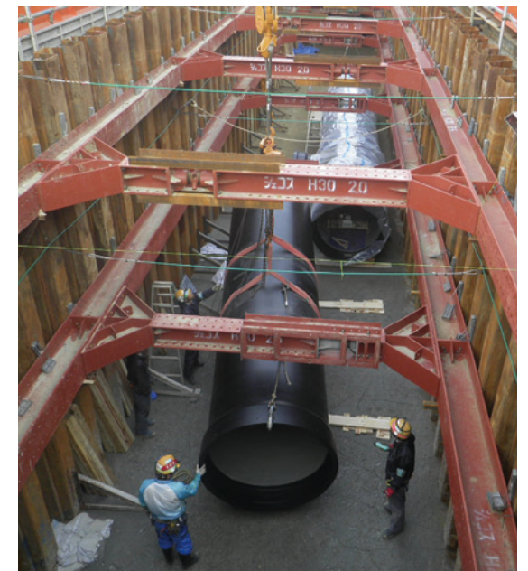
耐震管(ダクタイル鋳鉄管口径 1650mm)
