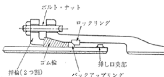
図 2.8 S II形鋳鉄管の接合
