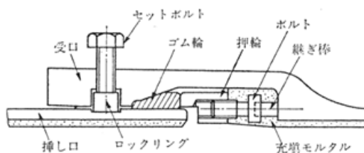
図 2.6 U F形鋳鉄管の接合
