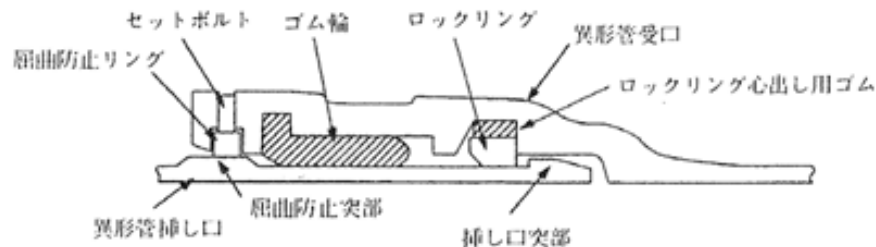
図 2.12 NS形铸铁管（異形管）の接合
