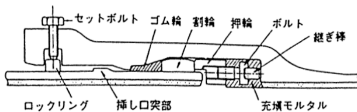
図 2.16 U S 形鋳鉄管 (S B 方式) の接合
